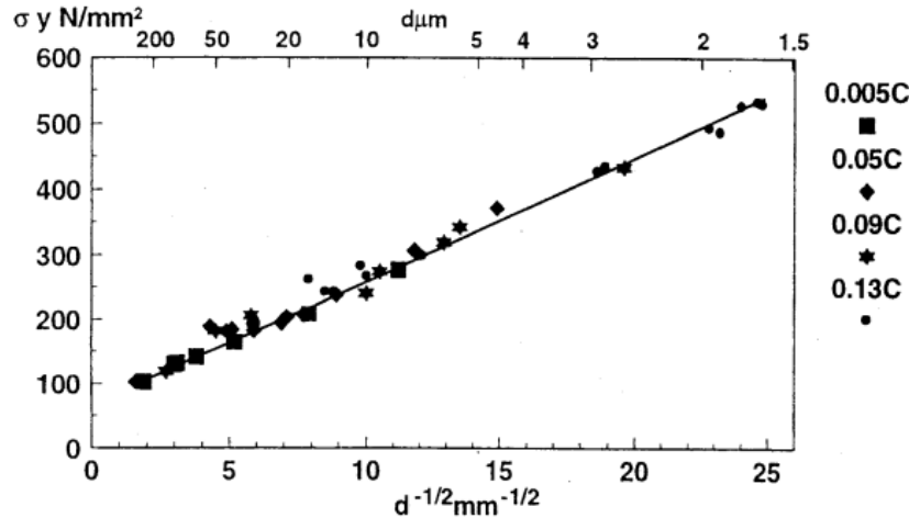
Figura 2 - Relação entre o limite de escoamento e o inverso da raiz quadrada do diâmetro do grão. (6)
