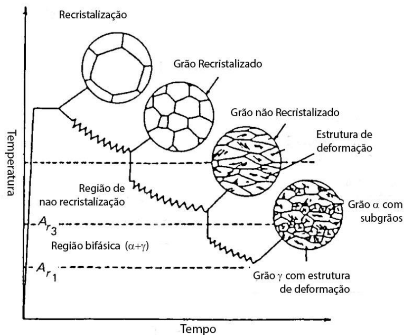
Figura 1 - Estágios da laminação controlada. (3)
