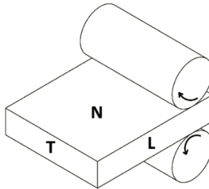
Figura 3 - Secções da chapa laminada adotadas para o estudo.
