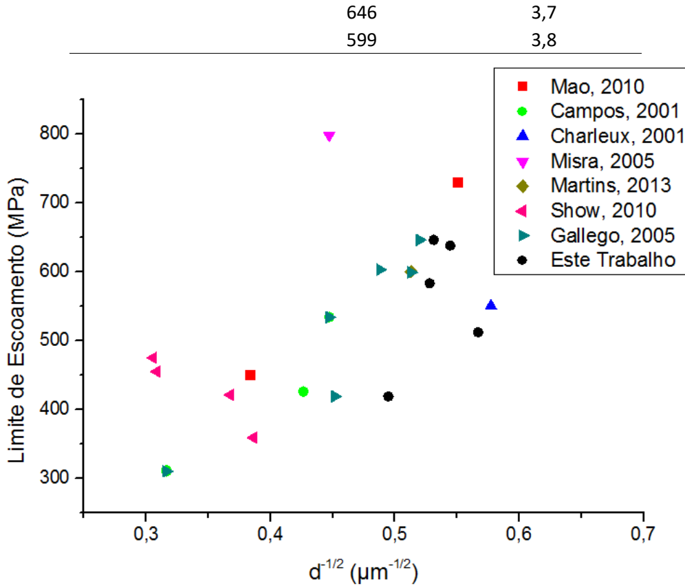
Figura 5 - Representação da relação de Hall-Petch para diversos materiais em comparação com os estudados. (9-15)
