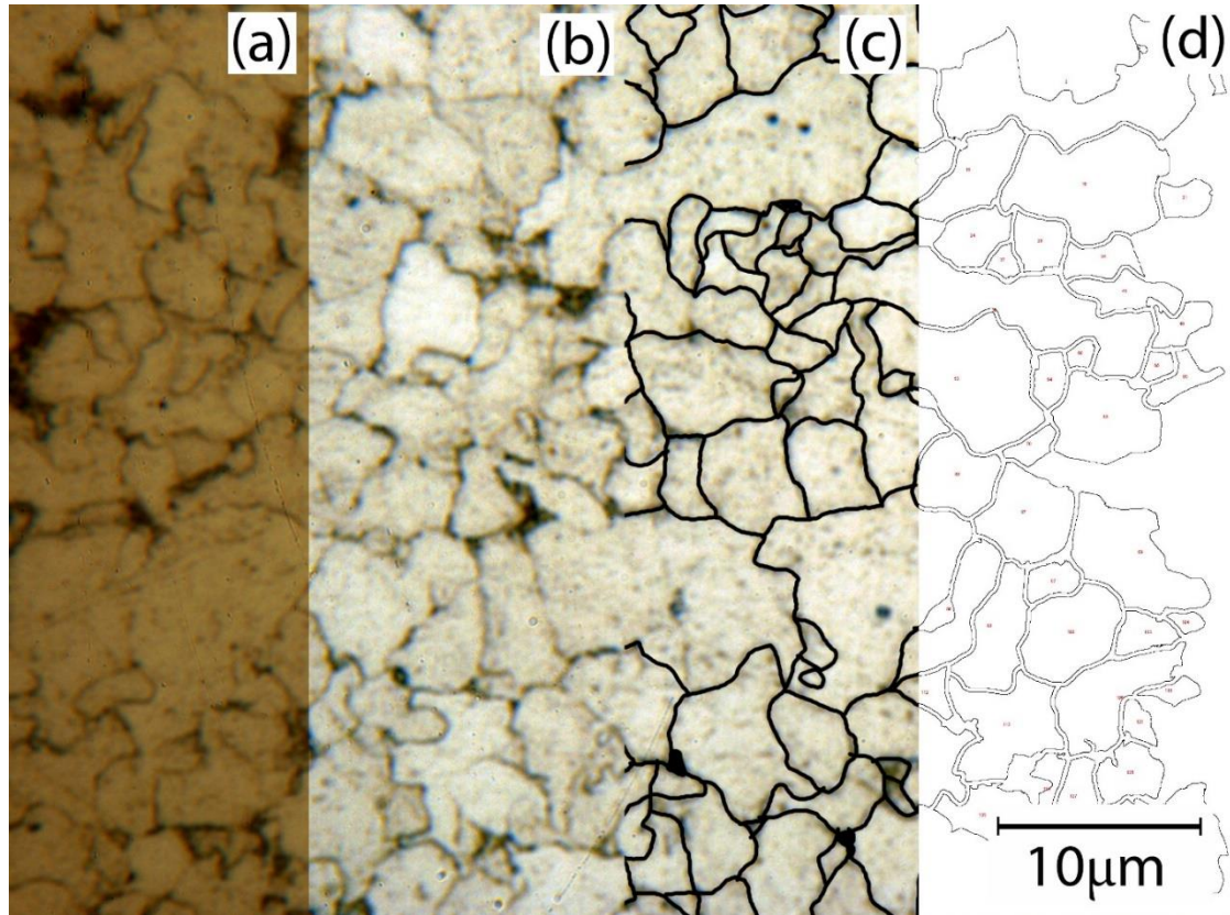
Figura 4 - Passos de tratamento das imagens. (a) Imagem original; (b) Imagem melhorada; (c) Contornos delineados; (d) Resultado de mapa de áreas no ImageJ.
