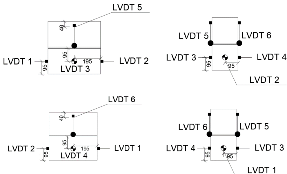
Figura 2 - Instrumentação Prismas
