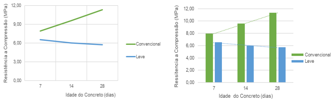
Figura 1- Resistência dos grautes
